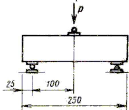
Схема испытания кирпича на изгиб
