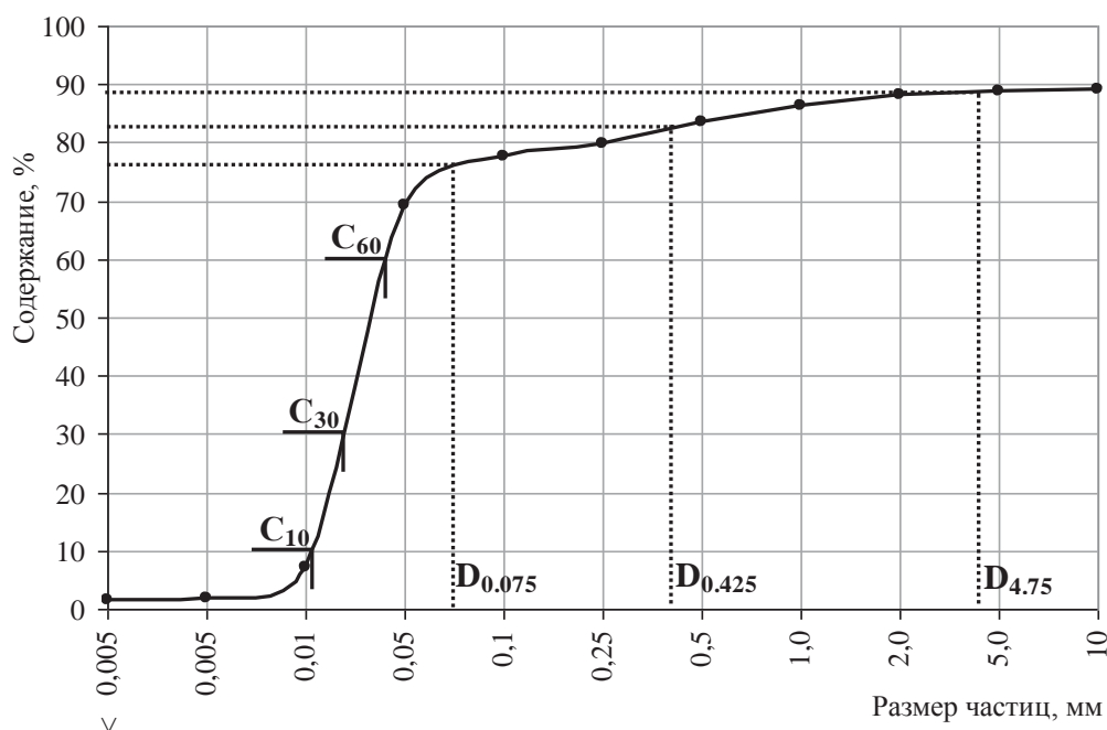
Рис. Е.1 Кумулятивная кривая гранулометрического состава
