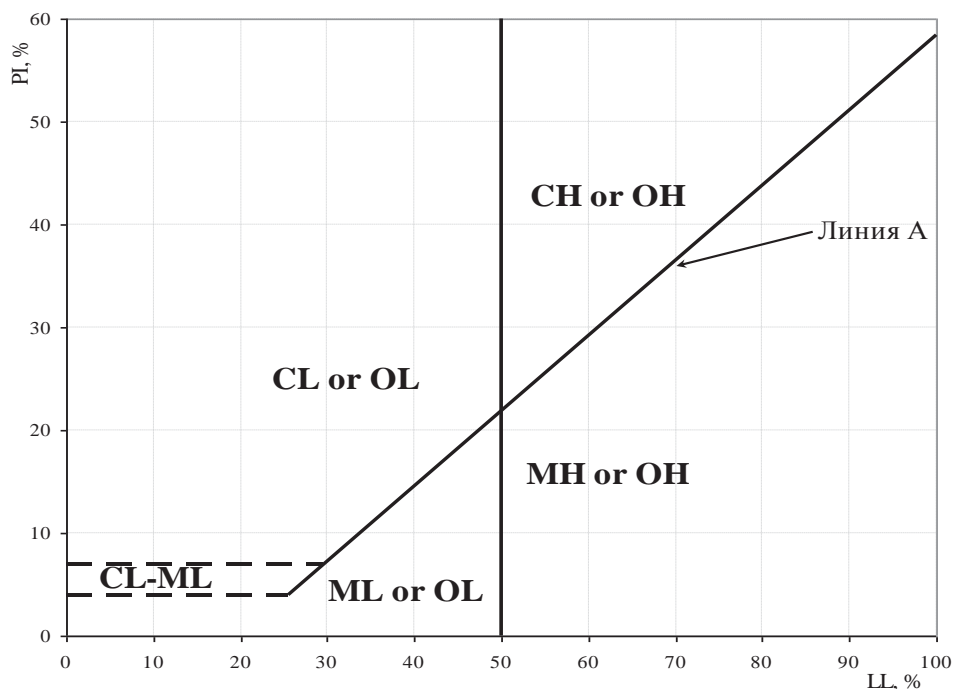
Рис. Е.2. График пластичности грунтов (Plasticity Chart).
